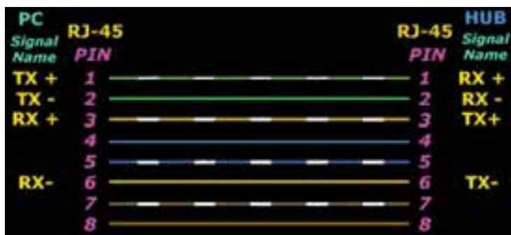
شکل ۴-۴۹- اتصالات کابل Straight برای کابل Cat5 با سرعت ۱۰ یا ۱۰۰ مگابیت بر ثانیه با استاندارد
